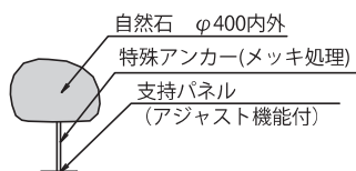
製品単体図
