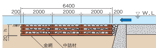
床止工断面図
