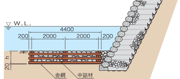
根固工断面図
