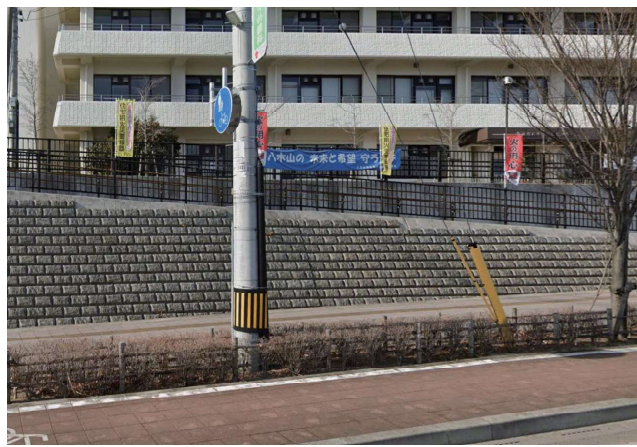
宮城県 仙台市役所 八木山市民センター 施工後12年
